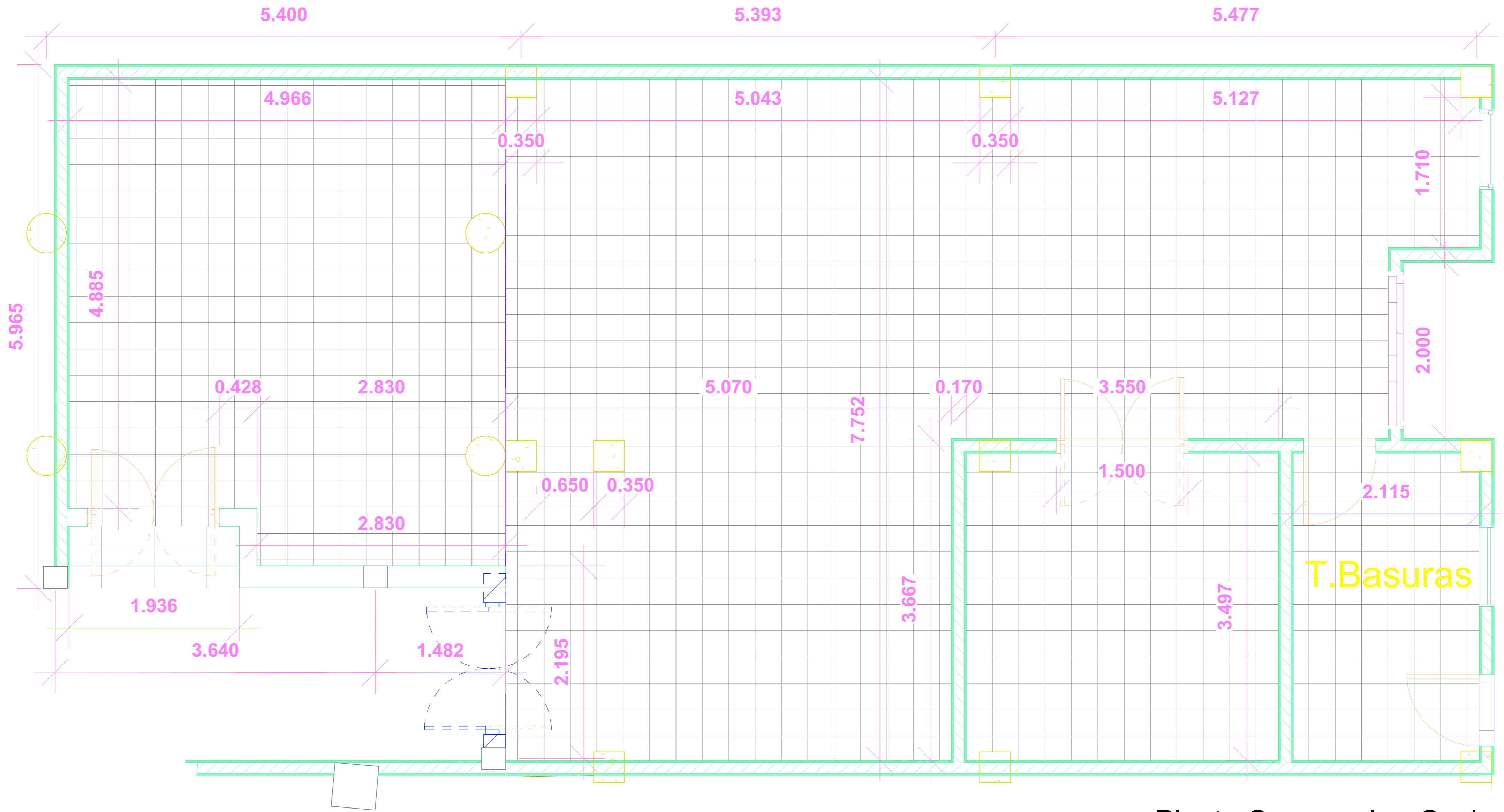
Planta Cenprende - Cocina Área Total 107.12 m 2 Escala 1:30
