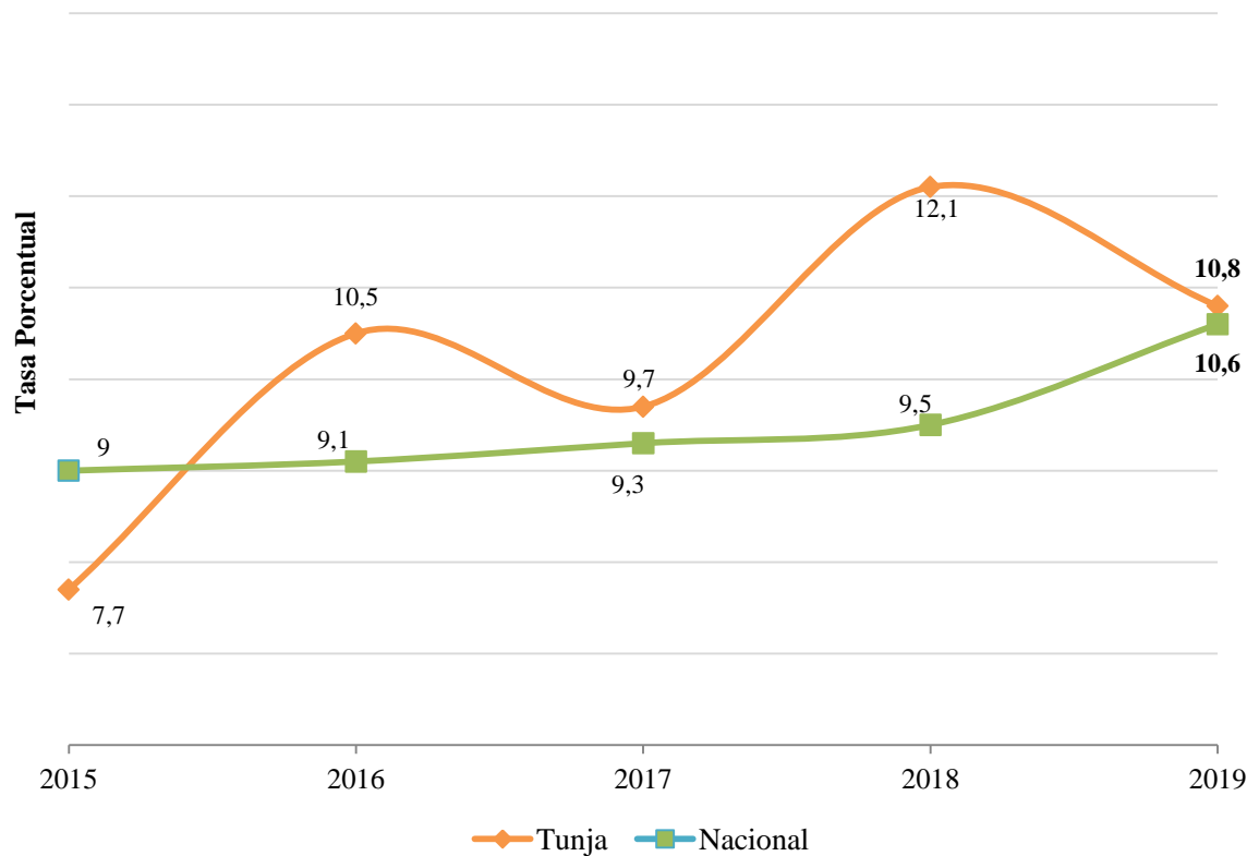
Gráfico 2: Tasa de Desempleo (TD) nacional y ciudad de Tunja
