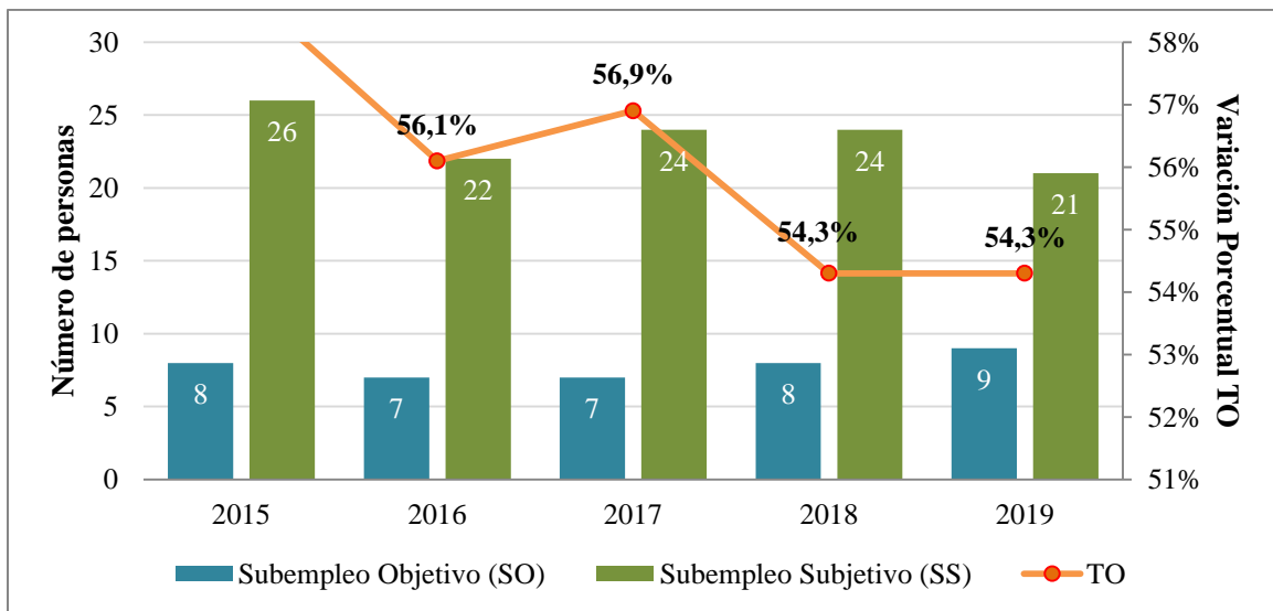
Gráfico 4: Subempleo Objetivo (SO) y Subempleo Subjetivo (SS) en Tunja. Trimestre móvil julio-septiembre (2015 - 2019).
